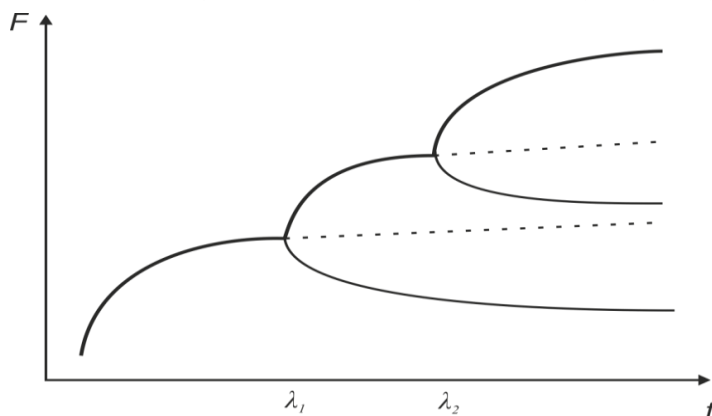
Рис. 5. Біфуркаційна модель
