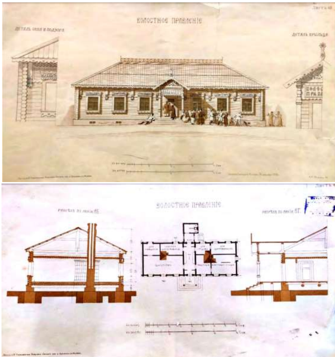
Фото 3, 4. План типового проєкту будівлі волосного правління.
