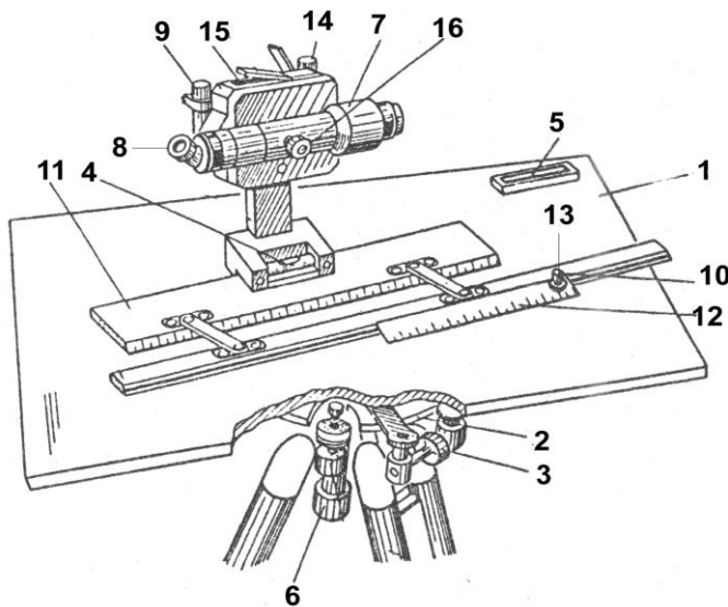
Рис. 8. Кіпрегель КН
