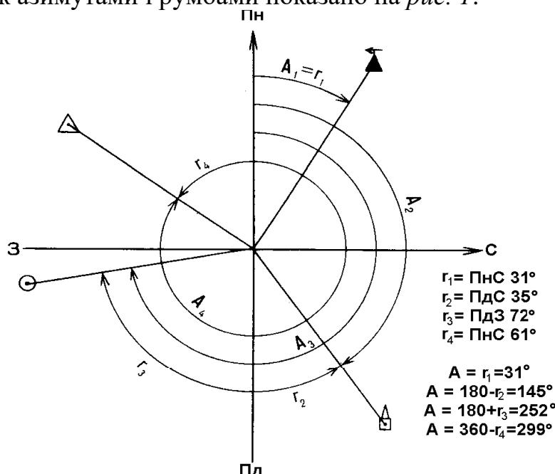
Рис. 1. Зв'язок між азимутами та дирекційними румбами
