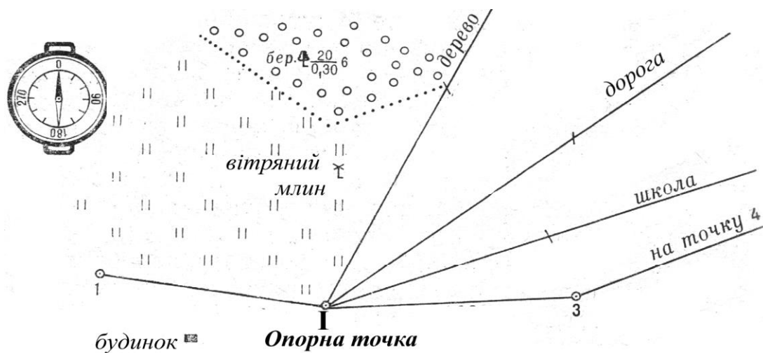
Рис. 10. Схема окомірної зйомки
