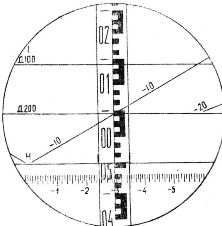
Рис. 9. Поле зору труби кіпрегеля КН
