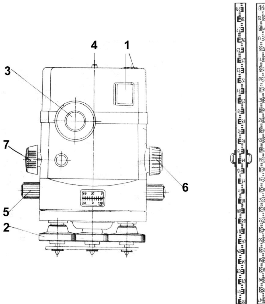
Рис. 5. Нівелір 2Н-10КЛ (а) та нівелірна рейка (б)
