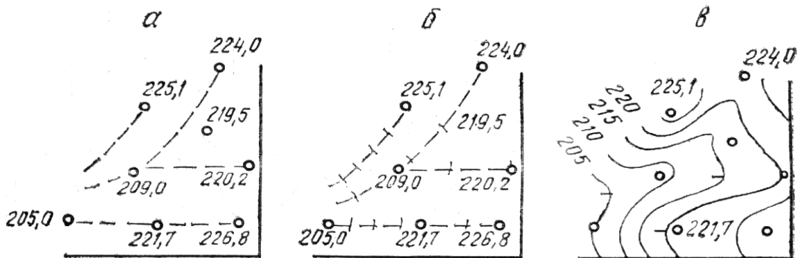
а) – напрямки структурних форм, б) – визначення положення горизонталей, в) – малювання горизонталей
