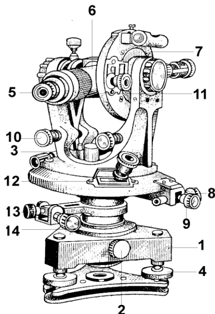
Рис. 3. Теодоліт ТТ-50
