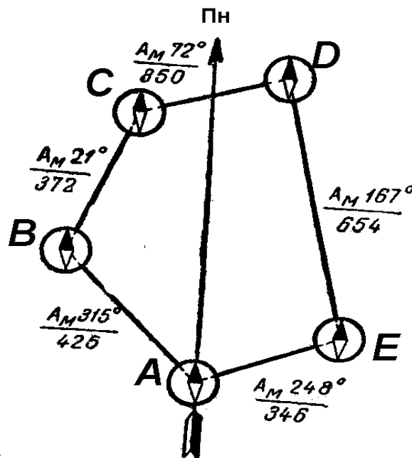
Рис. 12. Схема бусольного ходу
