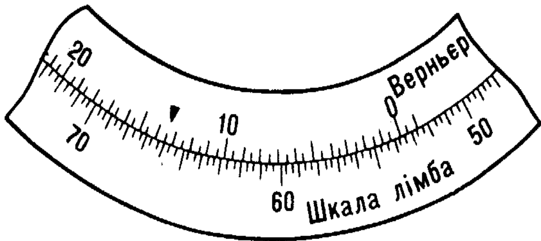
Рис. 4. Шкала лімба і верньєра
