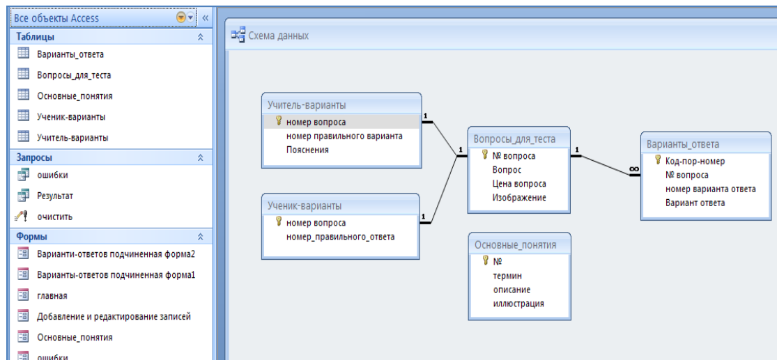
Рис. 1. Структура БД
